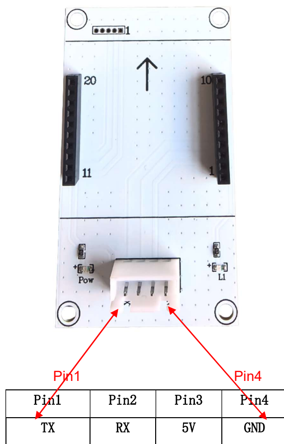
UART (TTL@115200bps)
